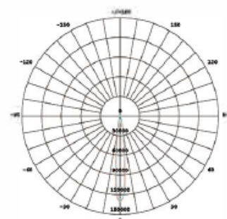
12D1908 Beam Angle(50%)12DEG
