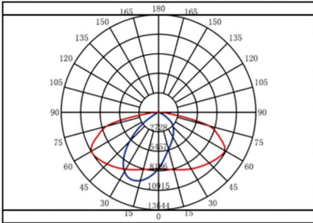
cd/klm — C0-C180, 151.8度 — C90-C270, 80.6度
